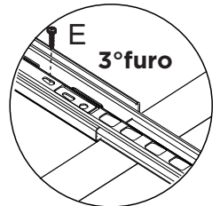
detalhe 3
