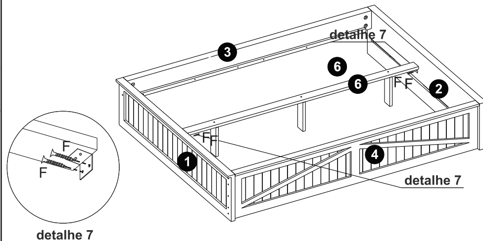
F- Parafuso ch ZB 3x16 (4x)
