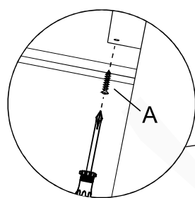
(8x) Parafusar em sentido horário.
