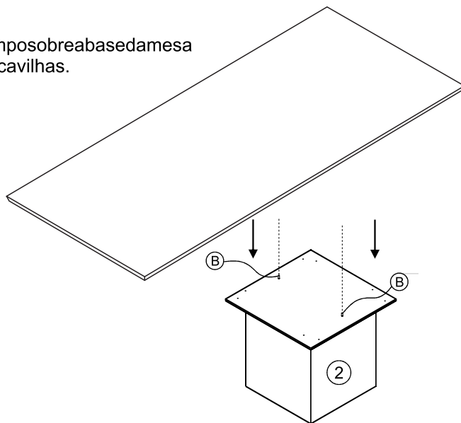
B-Cavilha Ø8x28(2x)
