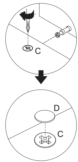
detalhe 5
