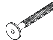
B- Parafuso ø7x60 (10x)
