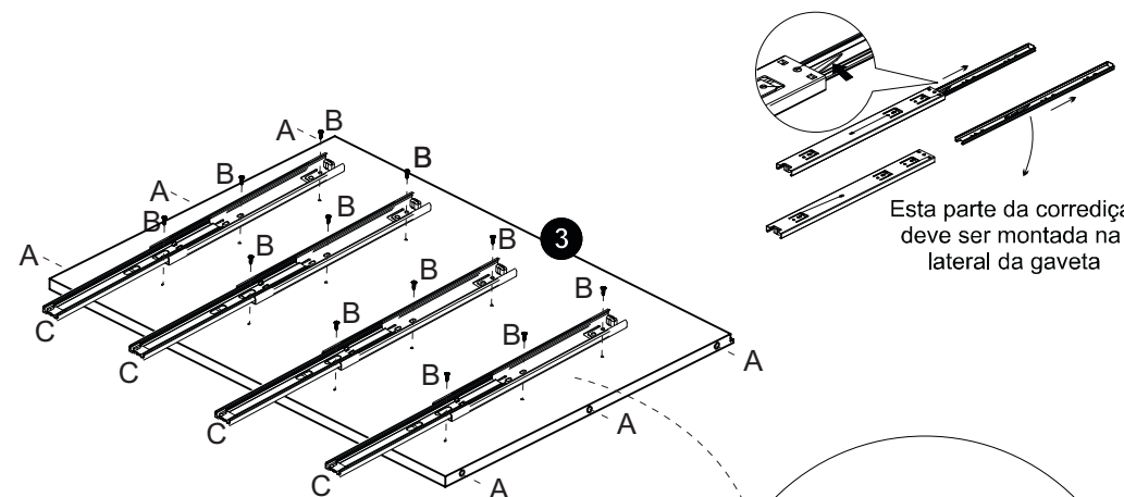
B - Parafuso 3.5x14 (24x)
